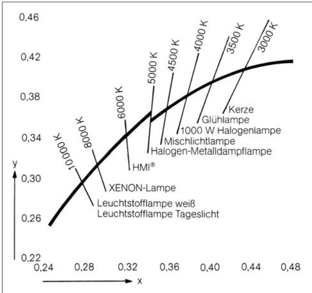
Ausschnitt aus der Normfarbtafel mit Planckschem Kurvenzug und Linien konstanter Farbtemperatur (Juddsche Geraden)
