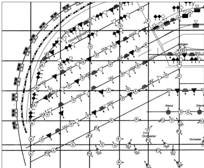
Ausschnitt aus einem Beleuchtungsplan einer AÜ-Fernsehproduktion
