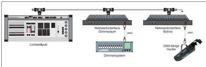
Grundlegender Aufbau eines 10Base2-Netzwerksystems mit linearer Netzwerktopologie
