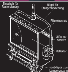
Kaltlicht Weichstrahler (220 W)
