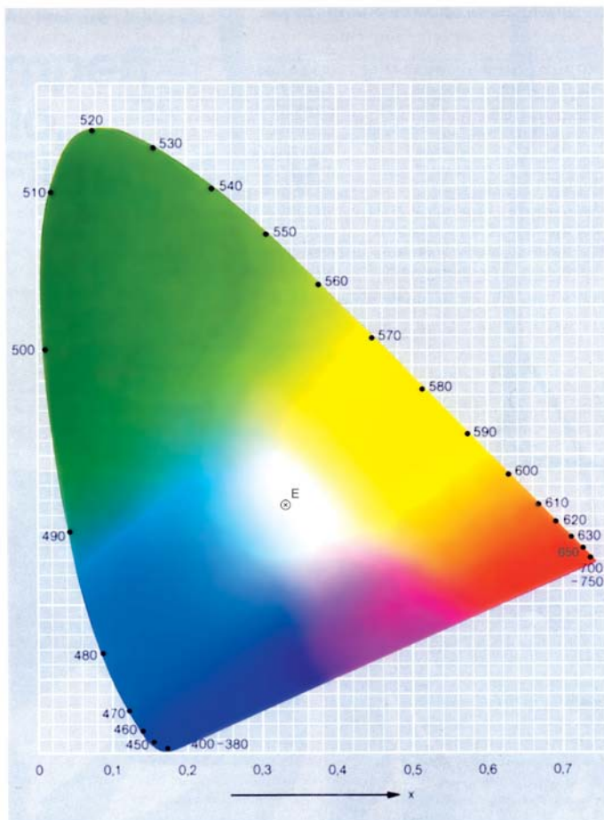
Normfarbtafel nach DIN 5033
