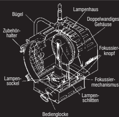
Stufenlinsenscheinwerfer 2kW
