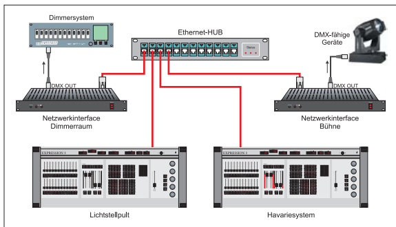
Grundlegender Aufbau eines 10BaseT-Netzwerksystems
