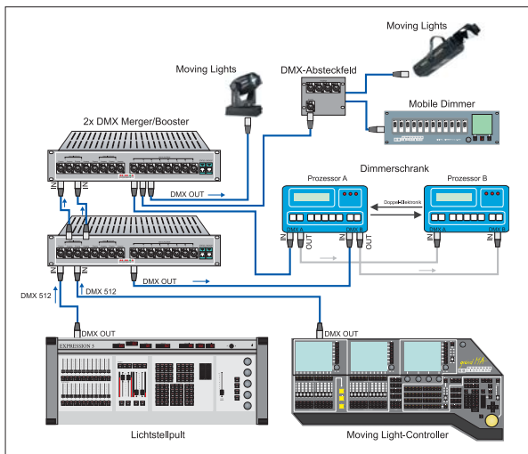
Aufbau einer Lichtanlage für Theater- oder Showproduktionen mit Lichtsteuerung, zusätzlicher Moving Light-Steuerung, Dimmersystem mit Doppel-Elektronik und DMX-Signalverteilung über DMX-Merger/Booster
