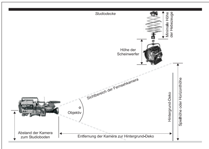
Berechnung der Spielhöhe als Kriterium bei der Ermittlung der erforderlichen Studiohöhe
