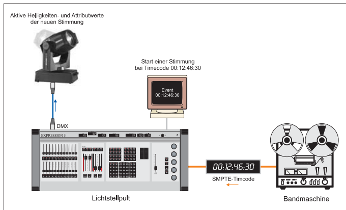
Einsatz des SMPTE-Timecodes zum automatisierten Abrufen gespeicherter Lichtstimmungen
