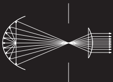
Strahlengang (Ellipsenspiegeloptik)
