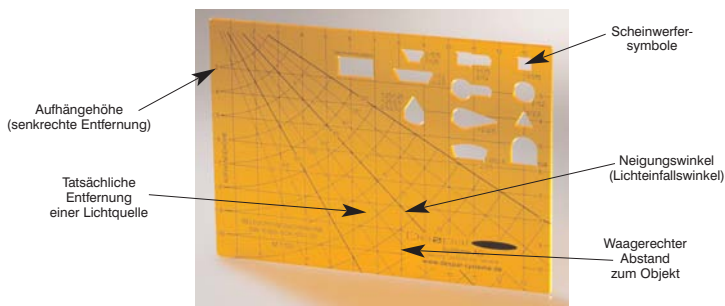
Beleuchtungsschablone gemäß DIN 15560 Teil 6, Maßstab 1:50
