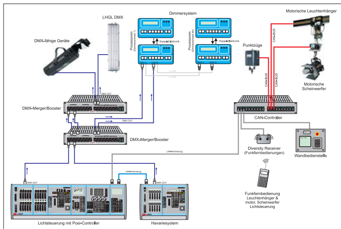
Aufbauschema einer Lichtanlage im Studio: Lichtsteuerung mit Posi-Controller, Havariesystem, Dimmersystem mit Doppel- und Dreielektronik, DMX-Signalverteilung über DMX-Merger/Booster und CAN-Bus für motorische Leuchtenhänger, Züge sowie Scheinwerfer
