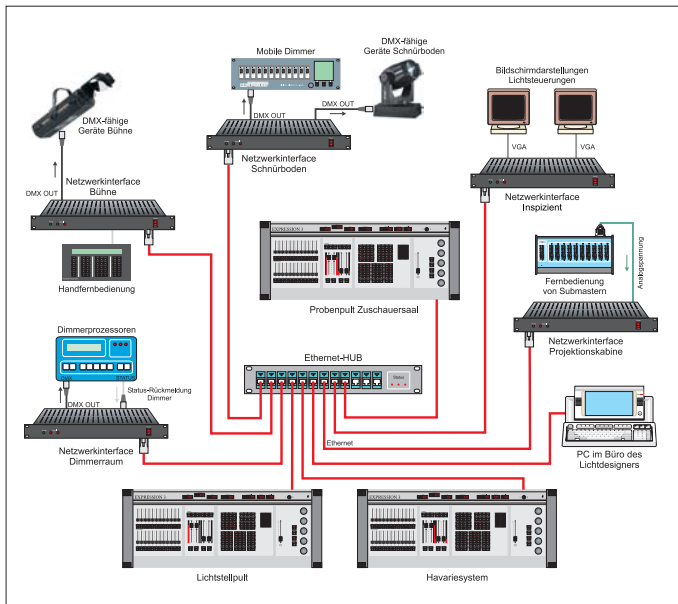
Aufbauschema einer Lichtanlage mit 10BaseT-Netzwerkinstallation im Theater: Lichtsteuerung, Havariesystem, Probenpult, Dimmersystem mit Status-Rückmeldung und STP-Netzwerkverkabelung
