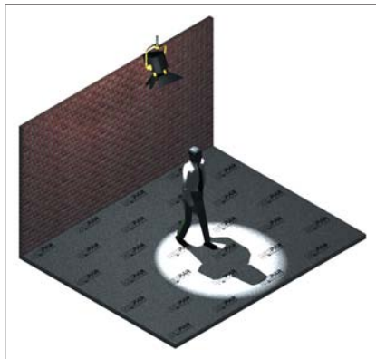
Schräg einfallendes Gegenlicht, Einfallswinkel 20°
