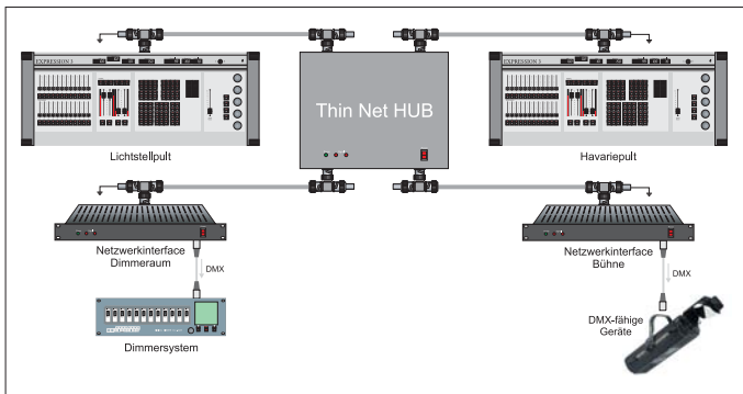
Grundlegender Aufbau eines 10Base2-Netzwerksystems mit sternförmiger Netzwerktopologie (an den einzelnen Segmenten können bis zu 28 weitere Geräte linear angeordnet werden)
