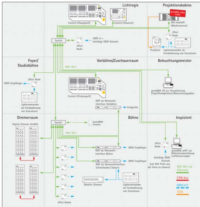
Aufbauschema einer Lichtanlage mit 10BaseT-Netzwerkinstallation im Theater: Lichtsteuerung, Havariesystem, Probenpult, Dimmersystem mit Status-Rückmeldung und STP-Netzwerkverkabelung
