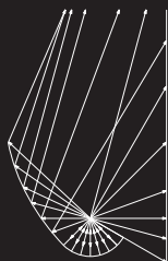
Strahlengang (asym. Reflektor)
